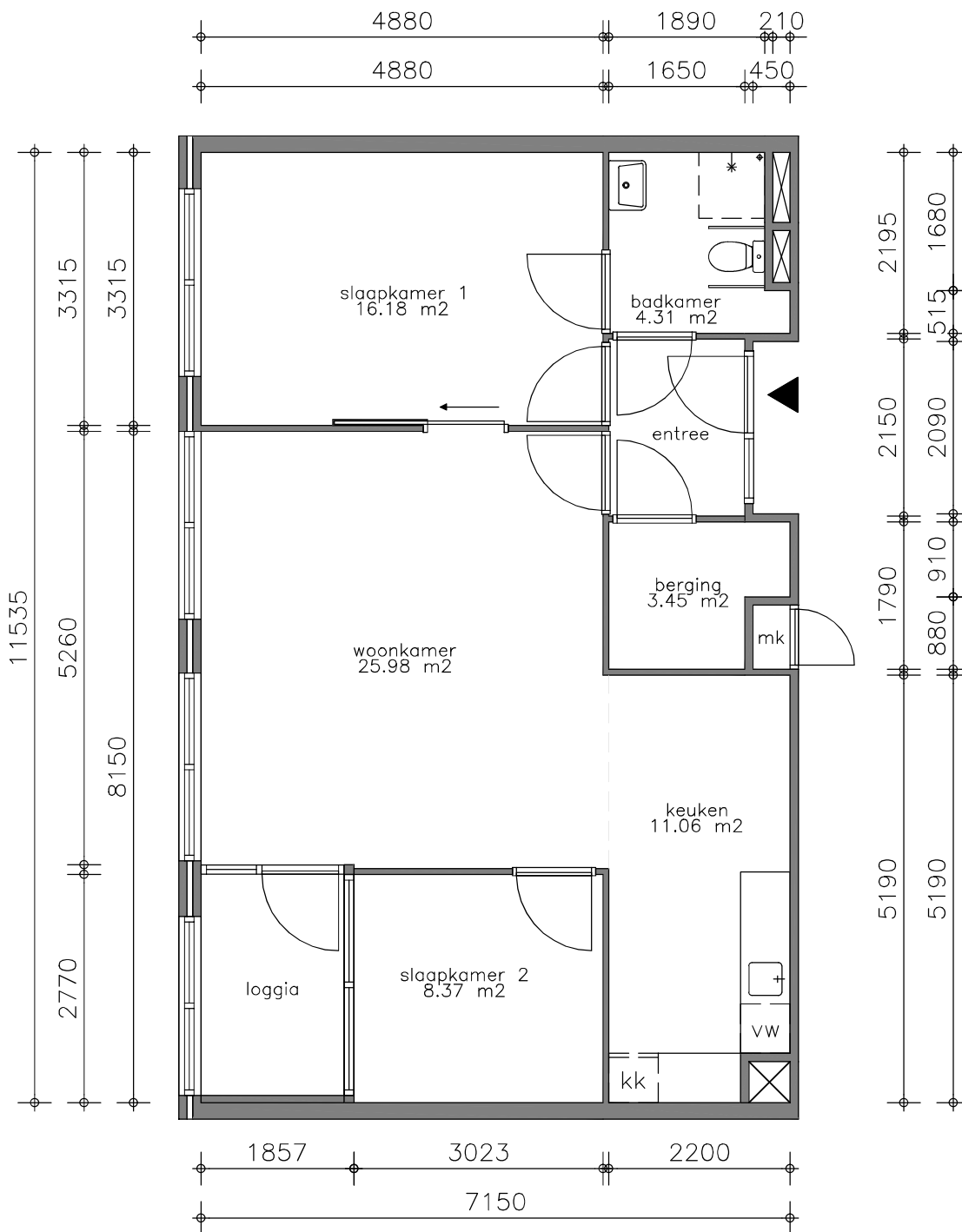
woonlaag 1
