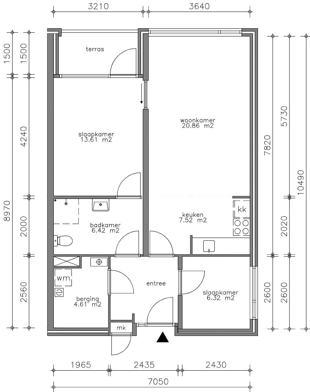
woonlaag 1
