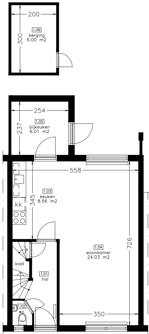
begane grond
