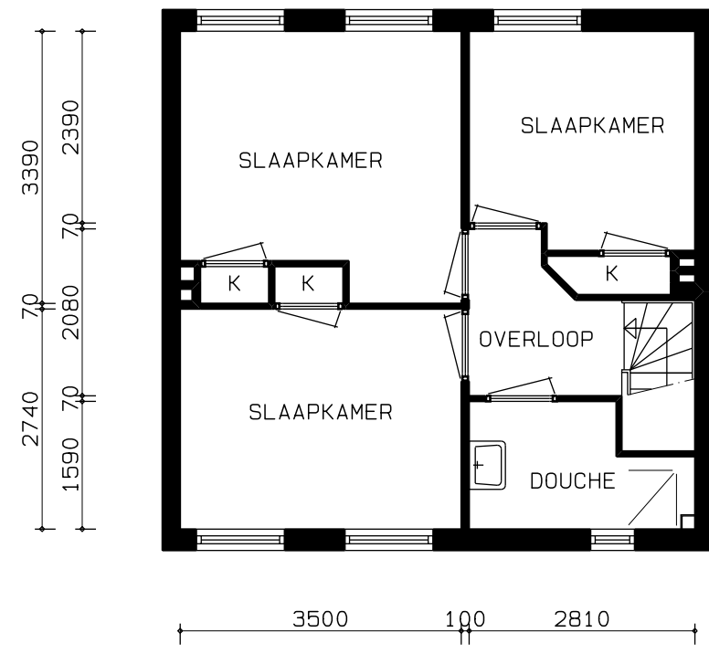
1E VERDIEPING
