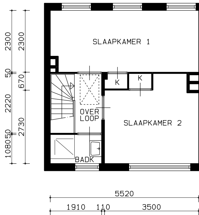
VERDIEPING
