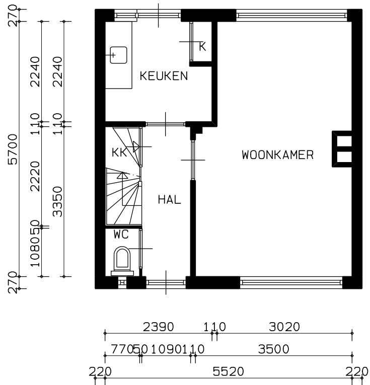
BEGANE GROND
